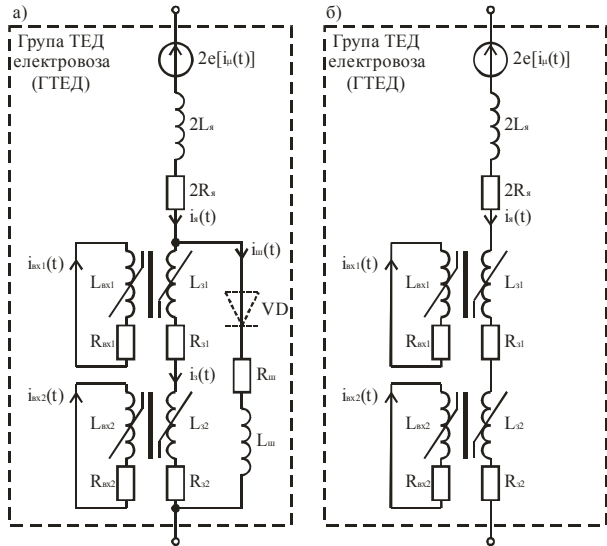
Рис. 2. Схема заміщення групи ТЕД ЕРС постійного струму: а – при послабленні збудження; б – при повному збудженні
