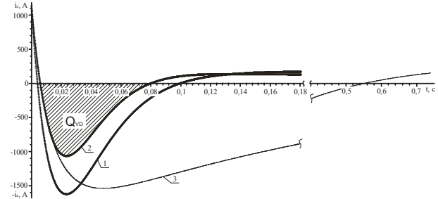
Рис. 6. Часові залежності генераторного струму електровозу, при різних схемах збудження ТЕД: 1 – ПП; 2 – ПЗЗ+VD; 3 – ПЗЗ
