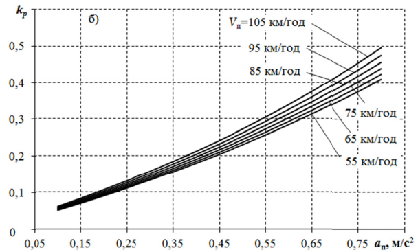
Рис. 1. Залежності k_p від пускового прискорення та пускової швидкості: а – колекторний привод; б – асинхронний привод
